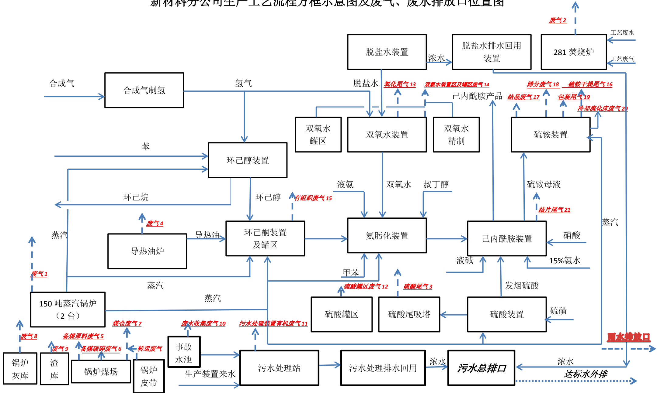
新材料分公司生产工艺流程方框示意图及废气、废水排放口位置图
